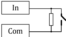
Під'єднання датчиків «Сухий контакт» з контролем обриву
