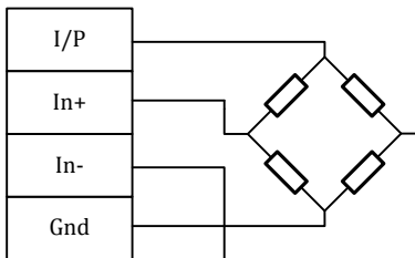
Подключение тензомота
